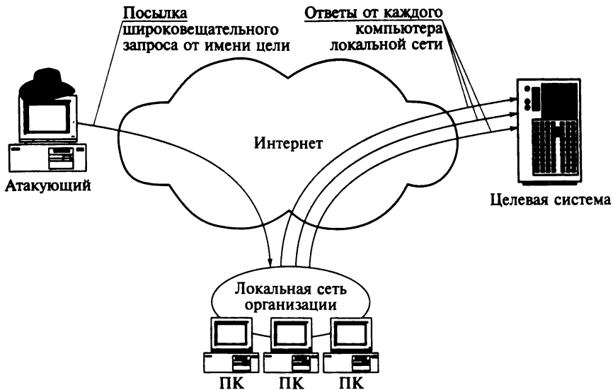
Рис. 3.7. Усиление атаки посылкой широковещательных запросов
