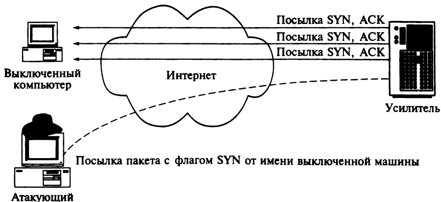
Рис. 3.8. Схема простого усиления атаки
