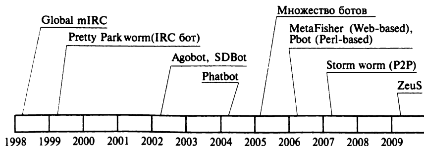
Рис. 3.3. Диаграмма появления сетей ботов
