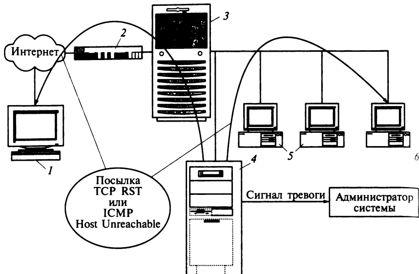
Рис. 5.19. Посылка пакета TCP Reset:
