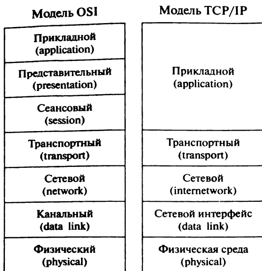
Рис. 1.1. Уровневые структуры стеков протоколов
