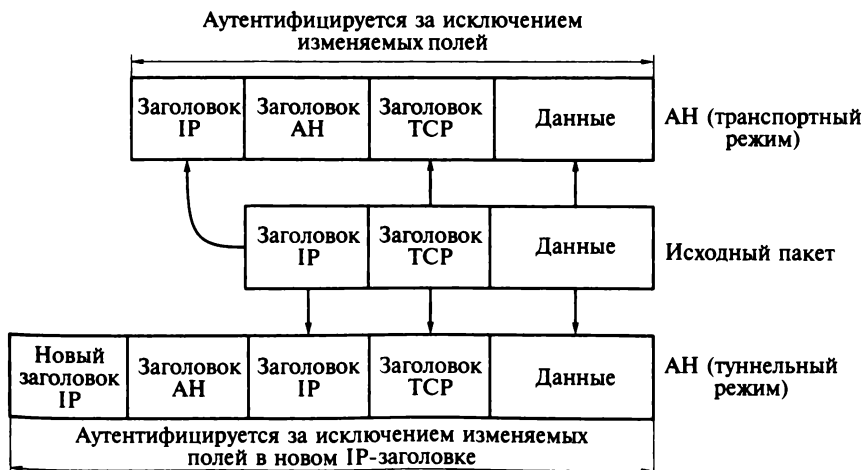
Рис. 6.6. Схема преобразования исходного пакета в АН-пакет
