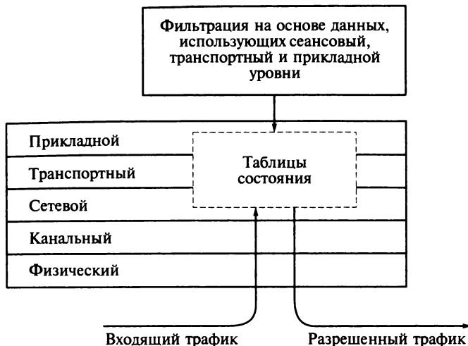
Рис. 4.9. Схема фильтрации при инспекции состояний
