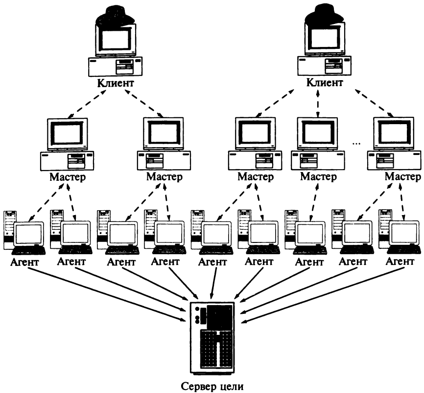
Рис. 3.4. Схема распределенной атаки «отказ в обслуживании»
