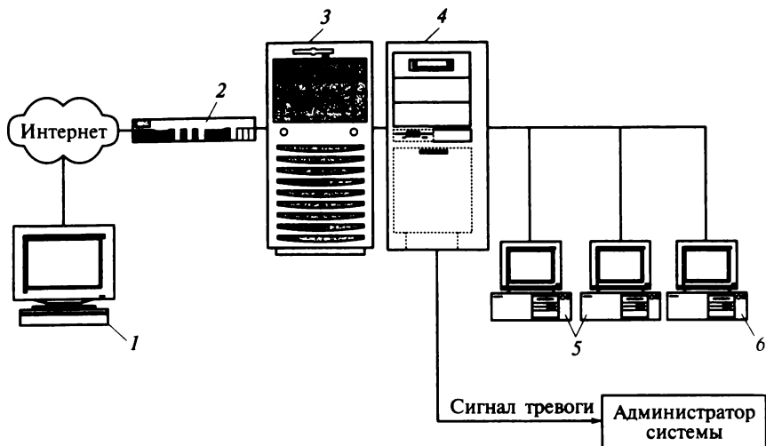
Рис. 5.21. Активная система предупреждения вторжений:
