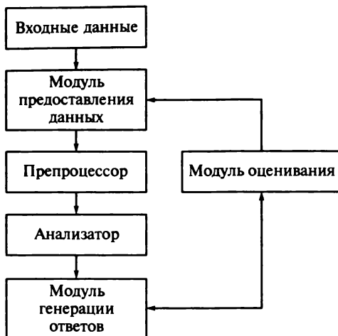
Рис. 5.13. Схема построения системы обучения без учителя
