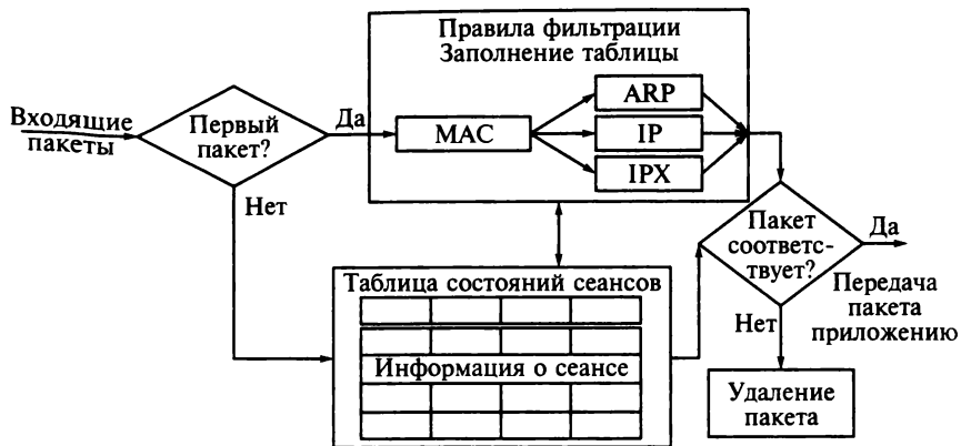
Рис. 4.12. Обработка пакетов в МЭ СППТ-2
