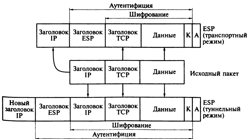
Рис. 6.8. Схема преобразования исходного пакета в пакет ESP
