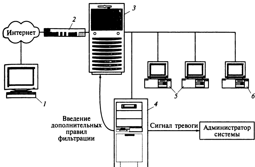
Рис. 5.20. Выдача сигнала фильтрующему устройству:
