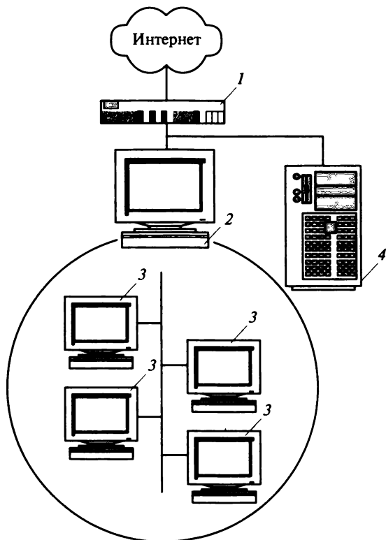
Рис. 5.15. Хост-приманка с серверами пользовательского уровня:
