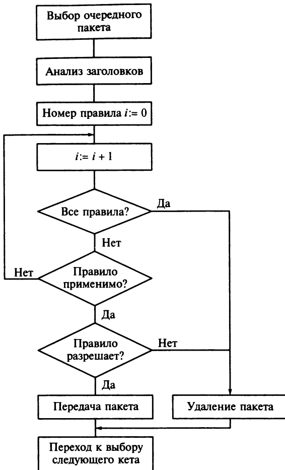
Рис. 4.4. Схема обработки пакетов при фильтрации
