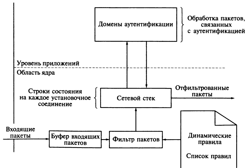
Рис. 4.8. Схема функционирования МЭ с динамической фильтрацией
